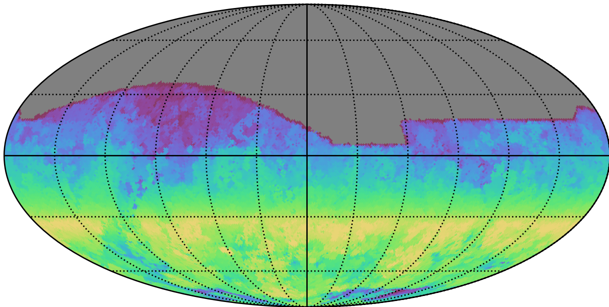
baseline_v3.3_10yrs All sky i band: AngleRange rotSkyPos
