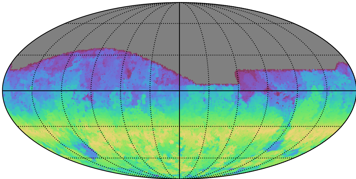
baseline_v3.3_10yrs All sky g band: AngleRange rotSkyPos
