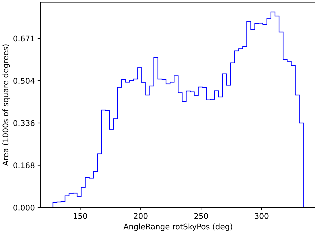
baseline_v3.3_10yrs All sky g band: AngleRange rotSkyPos
