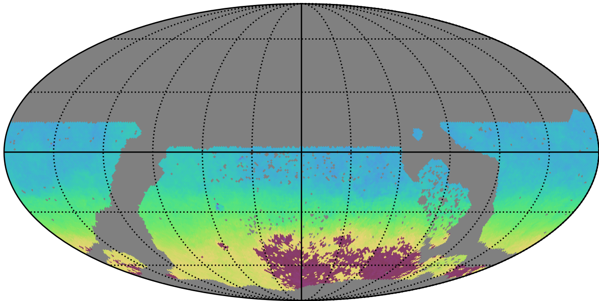
baseline_v3.3_10yrs WFD y band: AngleMean rotSkyPos
