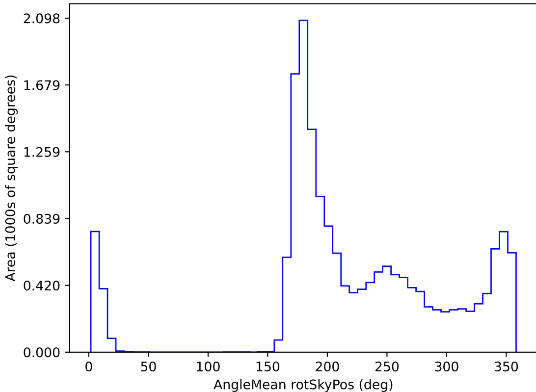
baseline_v3.3_10yrs WFD y band: AngleMean rotSkyPos
