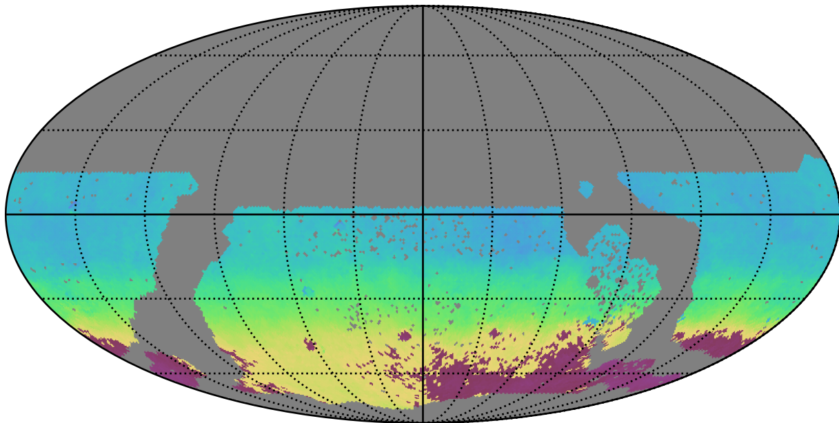
baseline_v3.3_10yrs WFD i band: AngleMean rotSkyPos
