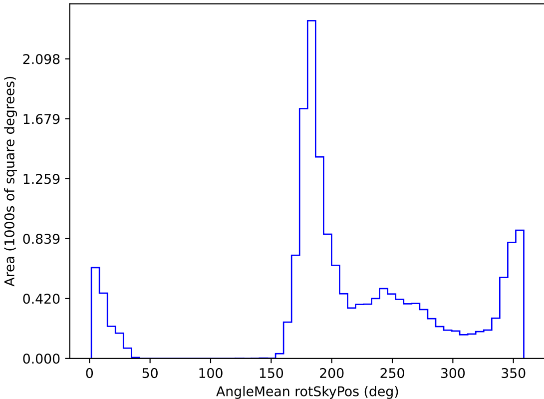
baseline_v3.3_10yrs WFD i band: AngleMean rotSkyPos
