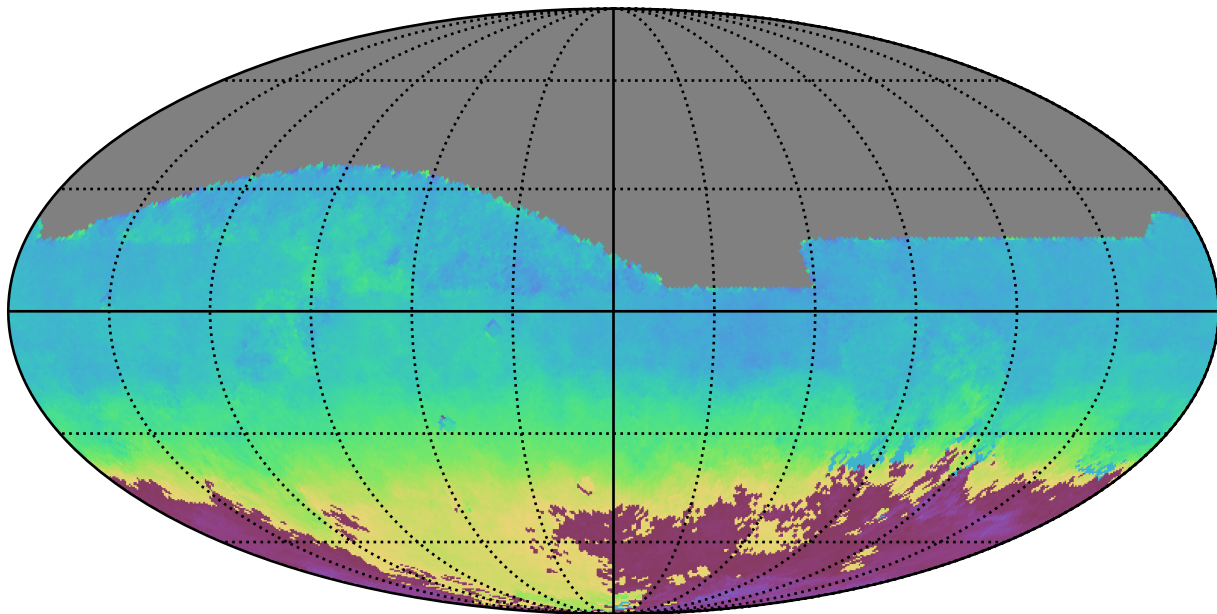
baseline_v3.3_10yrs All sky z band: AngleMean rotSkyPos
