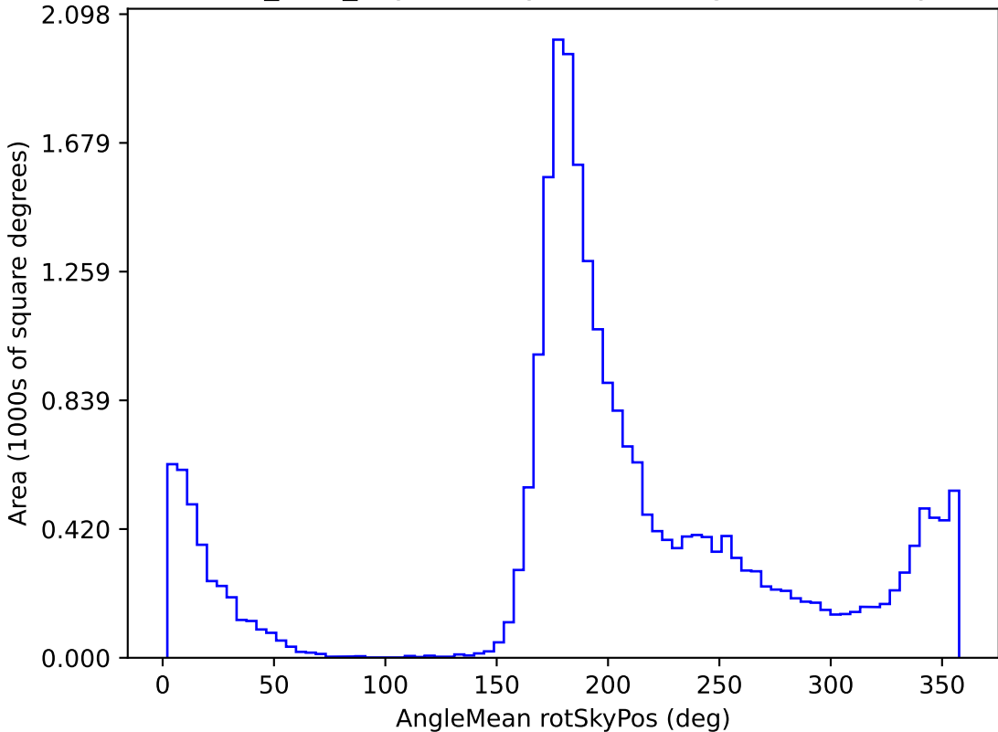
baseline_v3.3_10yrs All sky z band: AngleMean rotSkyPos
