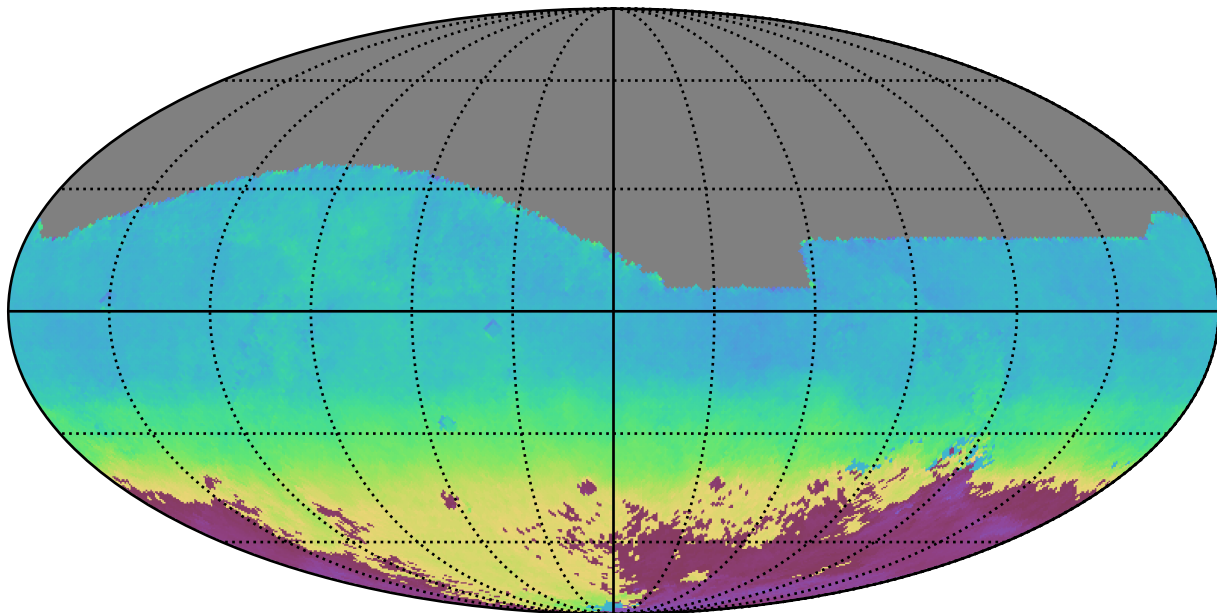
baseline_v3.3_10yrs All sky i band: AngleMean rotSkyPos
