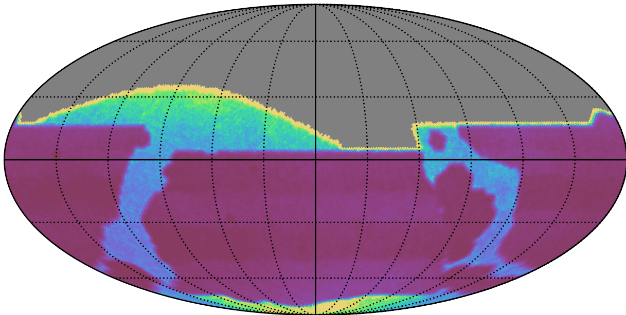
baseline_v3.3_10yrs : properMotion
