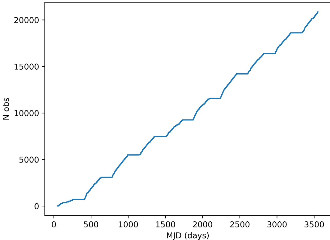
baseline_v3.3_10yrs note like DD:ELAISS1%: Cumulative
