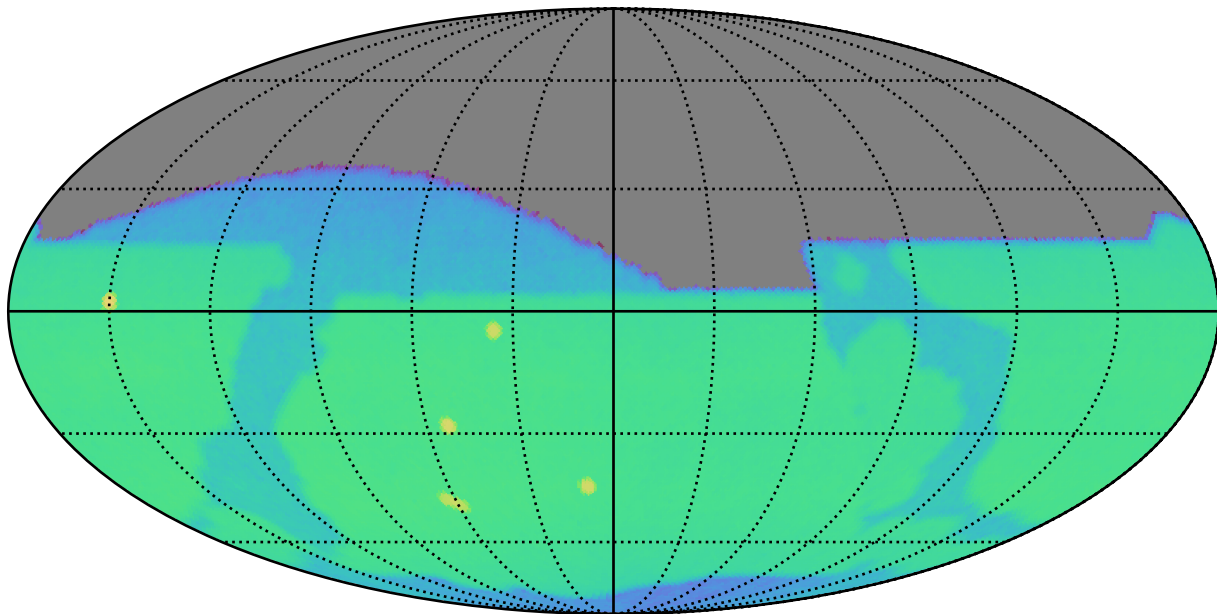
baseline_v3.3_10yrs z: CoaddM5
