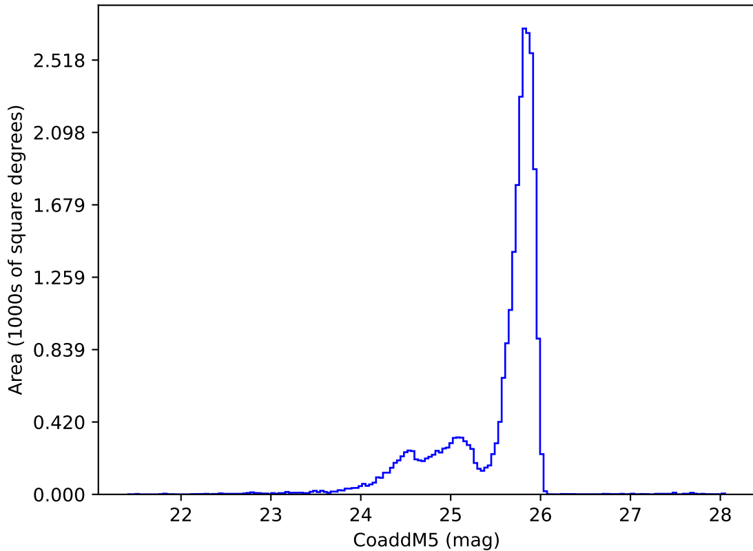
baseline_v3.3_10yrs z: CoaddM5
