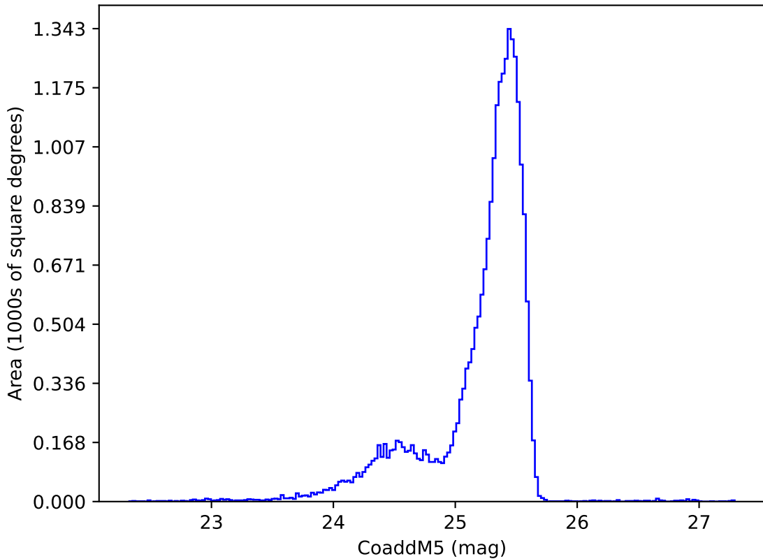
baseline_v3.3_10yrs u: CoaddM5
