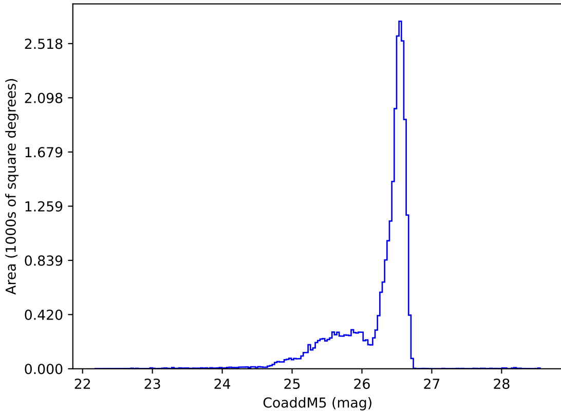
baseline_v3.3_10yrs i: CoaddM5
