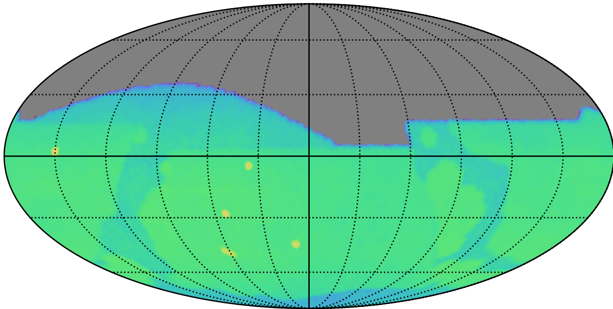
baseline_v3.3_10yrs g: CoaddM5
