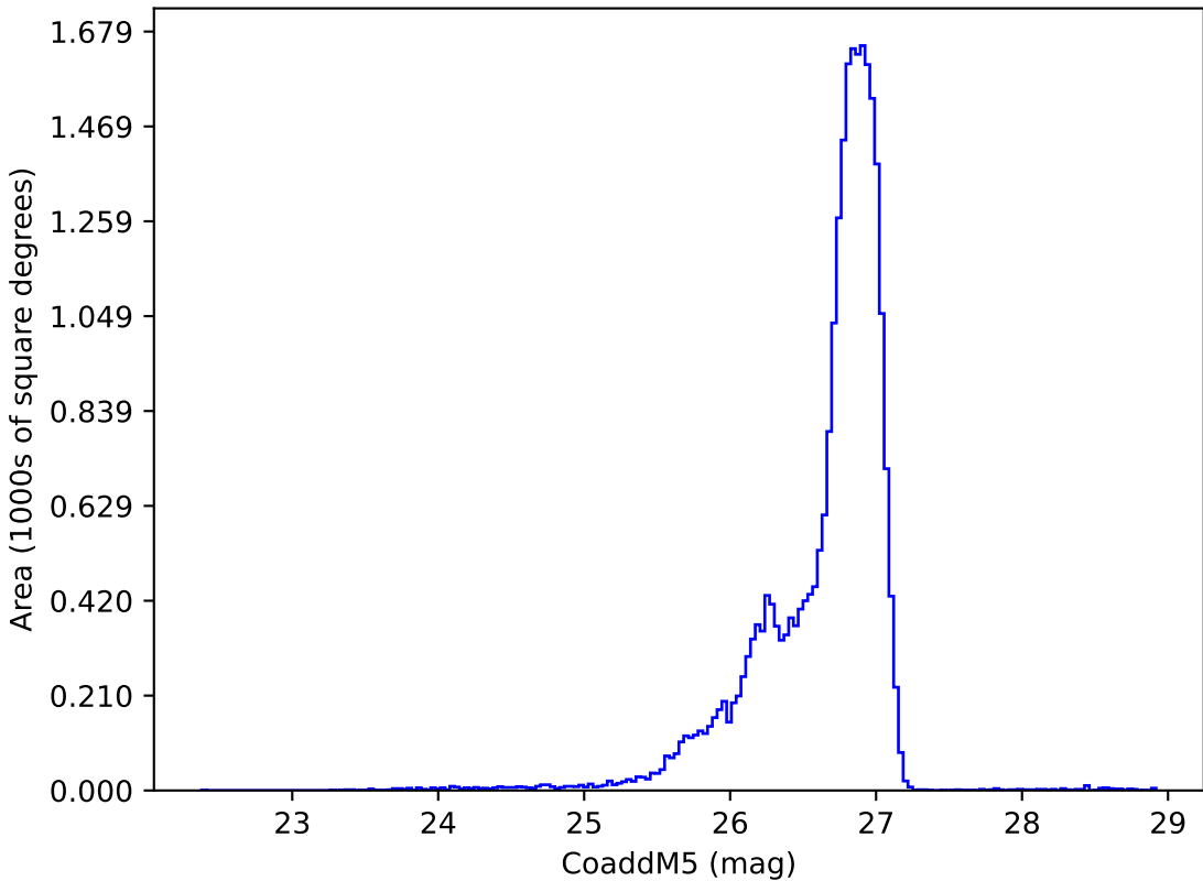
baseline_v3.3_10yrs g: CoaddM5
