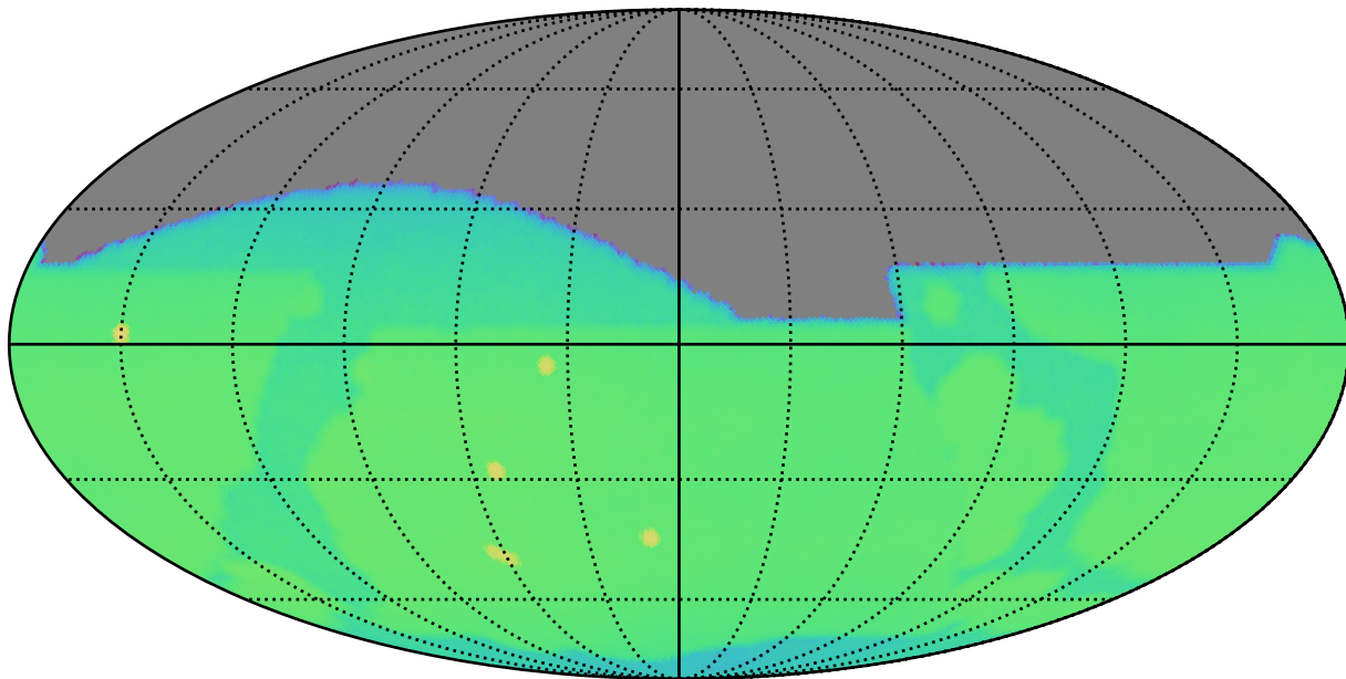
baseline_v3.3_10yrs : CoaddM5
