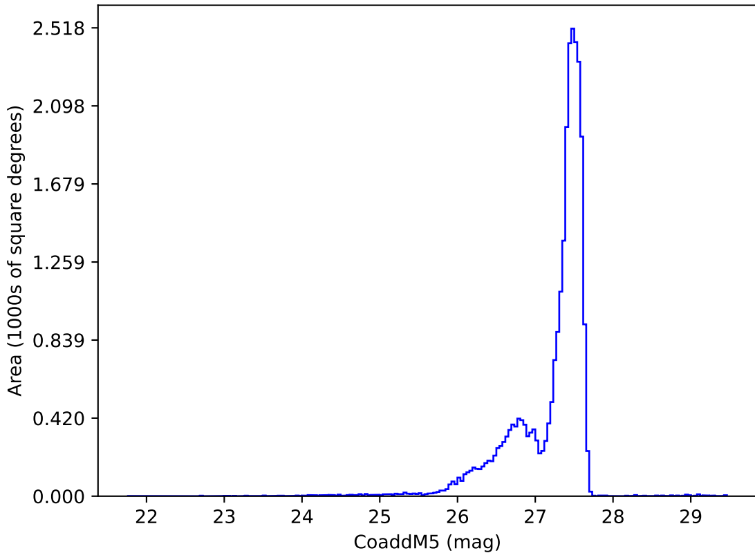
baseline_v3.3_10yrs : CoaddM5
