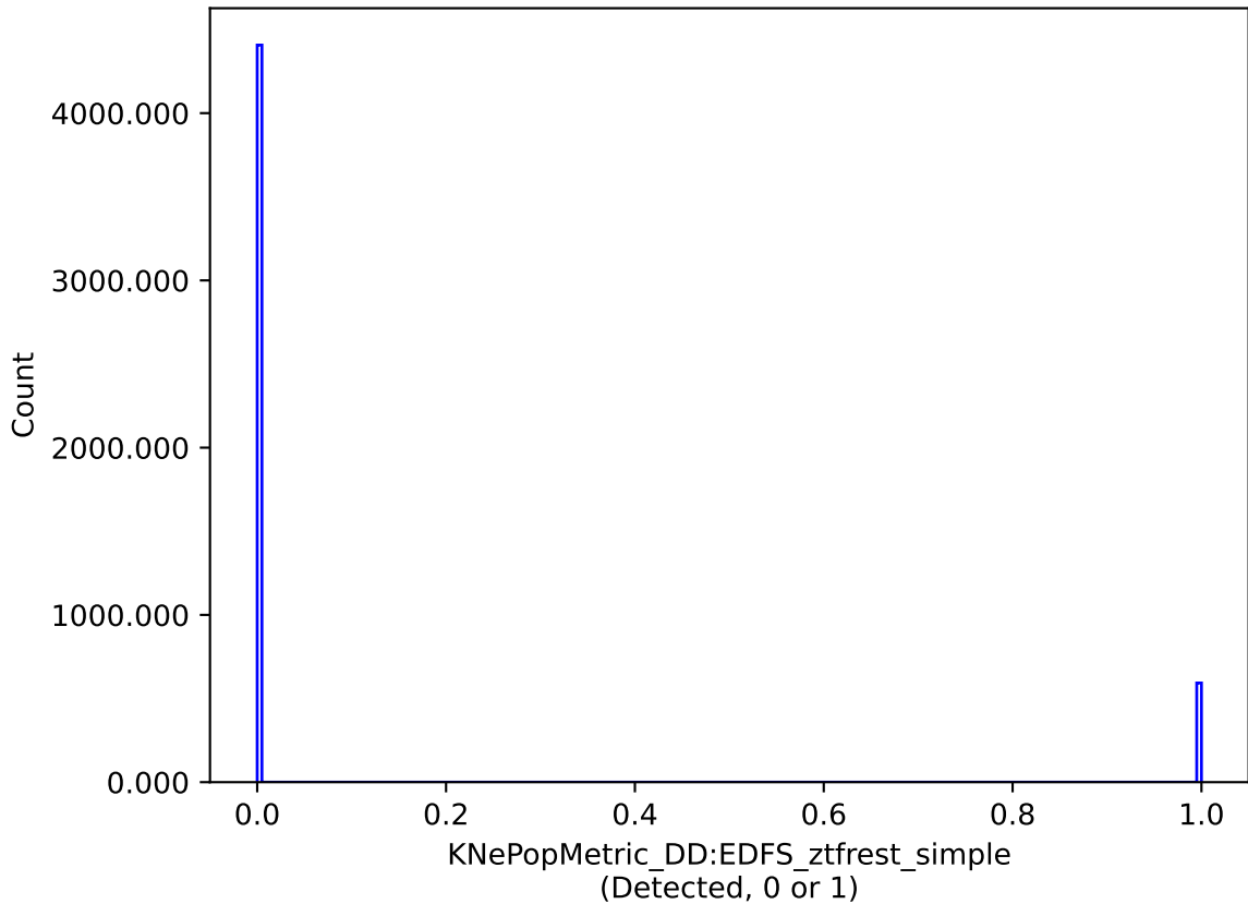
baseline_v3.3_10yrs DD:EDFS: KNePopMetric_DD:EDFS_ztfrest_simple
