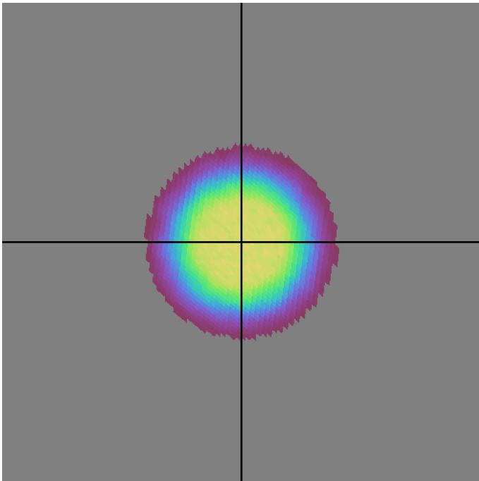
baseline_v3.3_10yrs r band: DD:ELAISS1 NVisits
