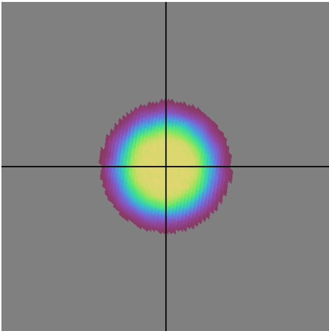
baseline_v3.3_10yrs all bands: DD:ELAISS1 NVisits
