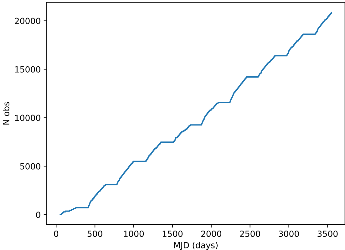
baseline_v3.3_10yrs all bands: DD:ELAISS1 Cumulative NVisits
