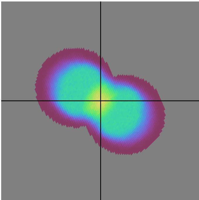
baseline_v3.3_10yrs z band: DD:EDFS NVisits
