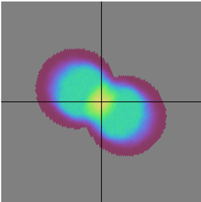
baseline_v3.3_10yrs r band: DD:EDFS NVisits
