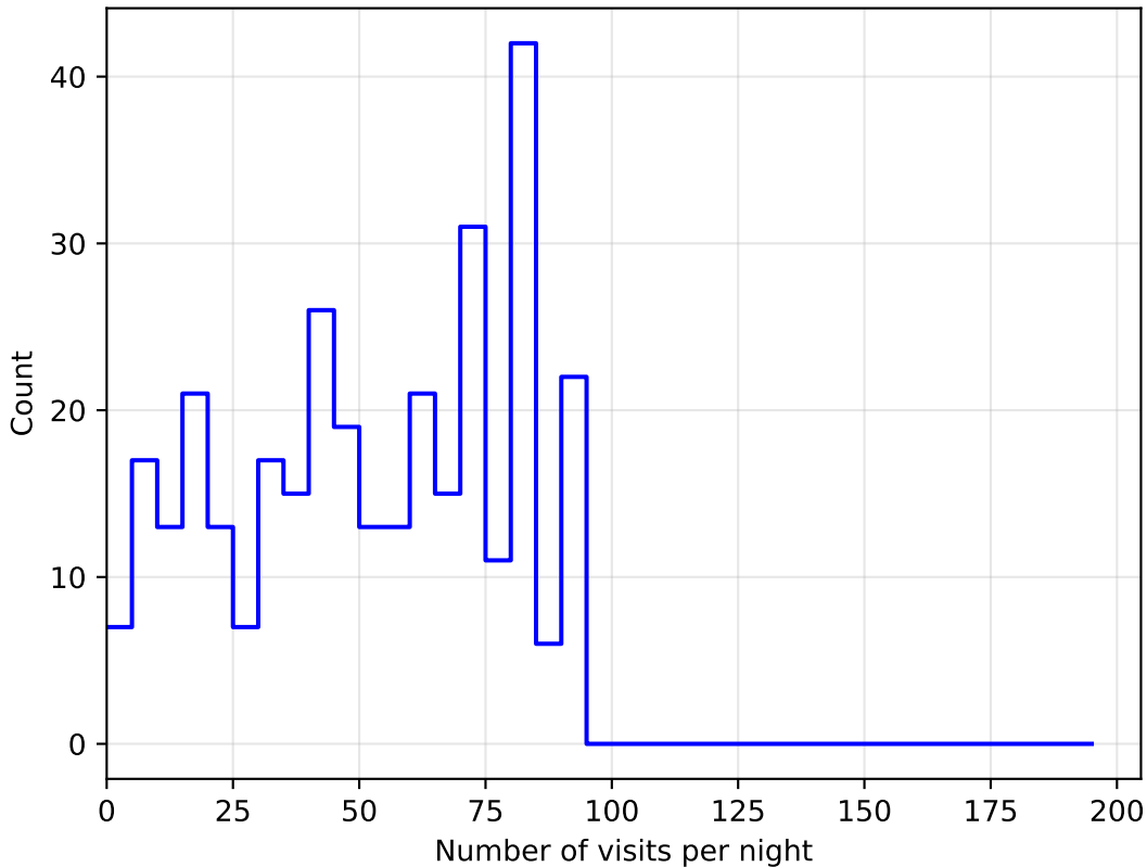
baseline_v3.3_10yrs all bands: DD:EDFS NVisitsPerNight
