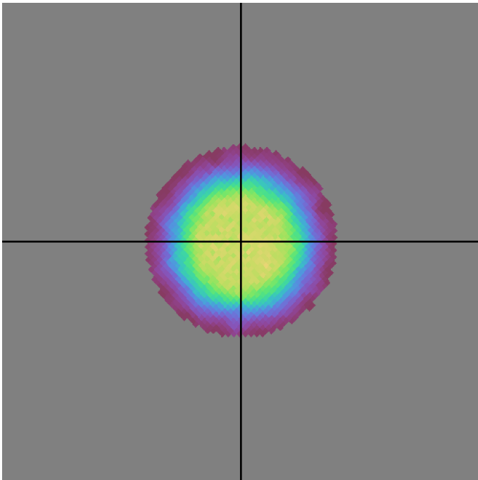
baseline_v3.3_10yrs y band: DD:ECDFS NVisits
