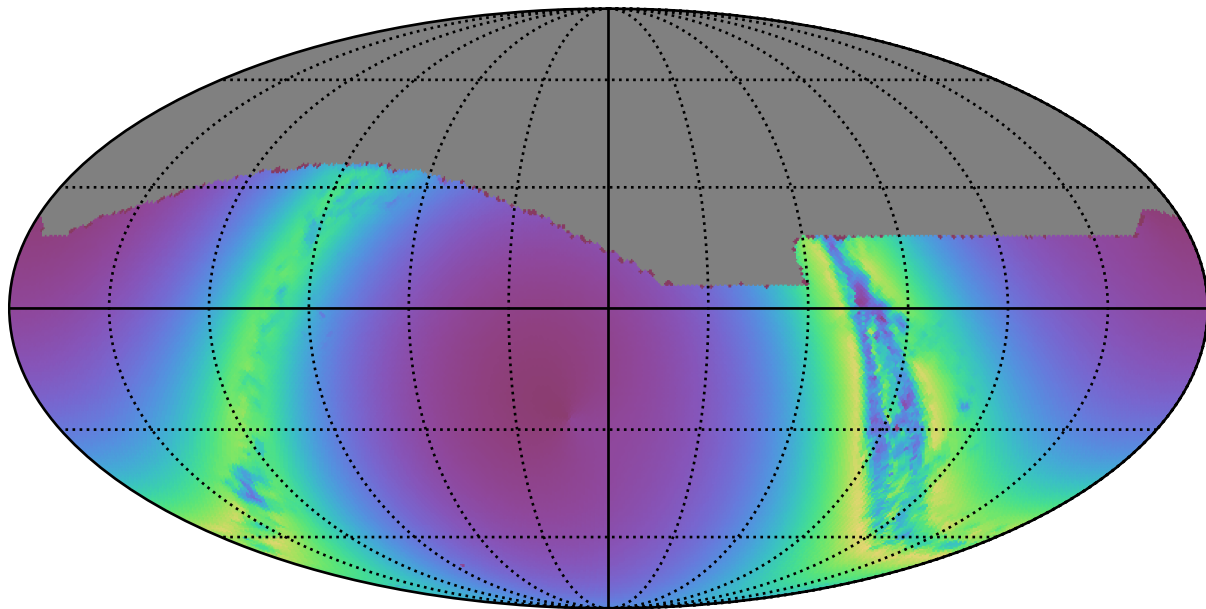
baseline_v3.2_10yrs : young_stars
