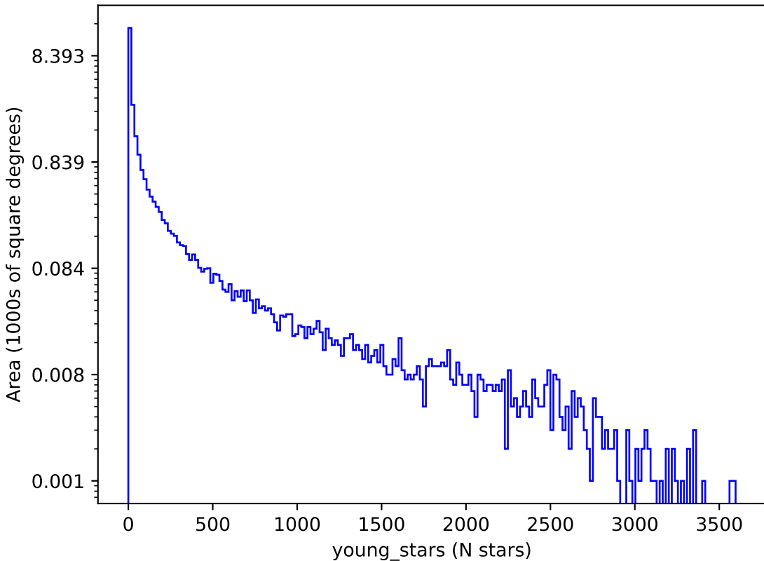
baseline_v3.2_10yrs : young_stars
