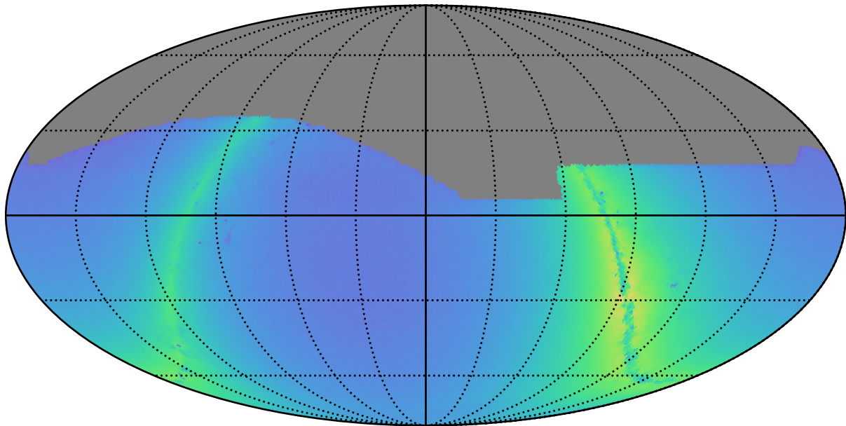
baseline_v3.2_10yrs i: Nstars_no_crowding
