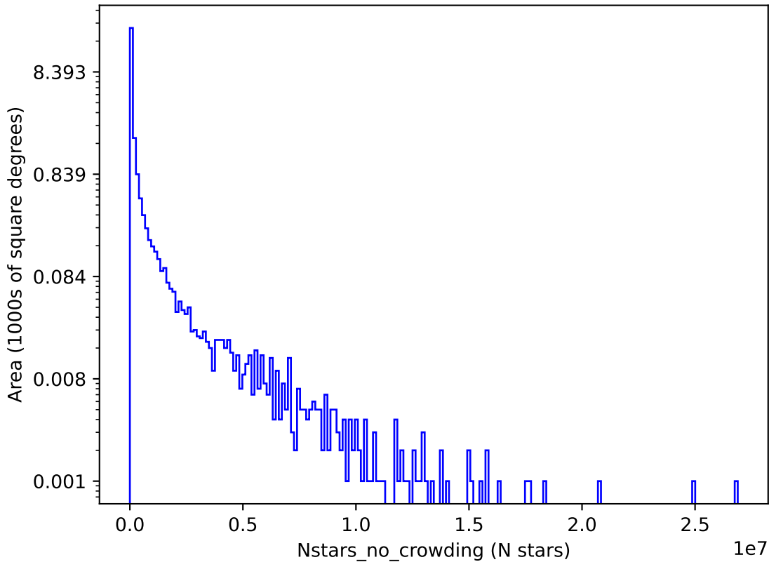
baseline_v3.2_10yrs i: Nstars_no_crowding
