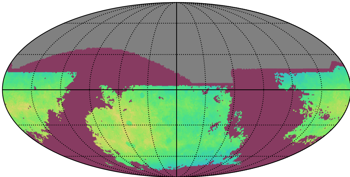
baseline_v3.2_10yrs i: NgalScale
