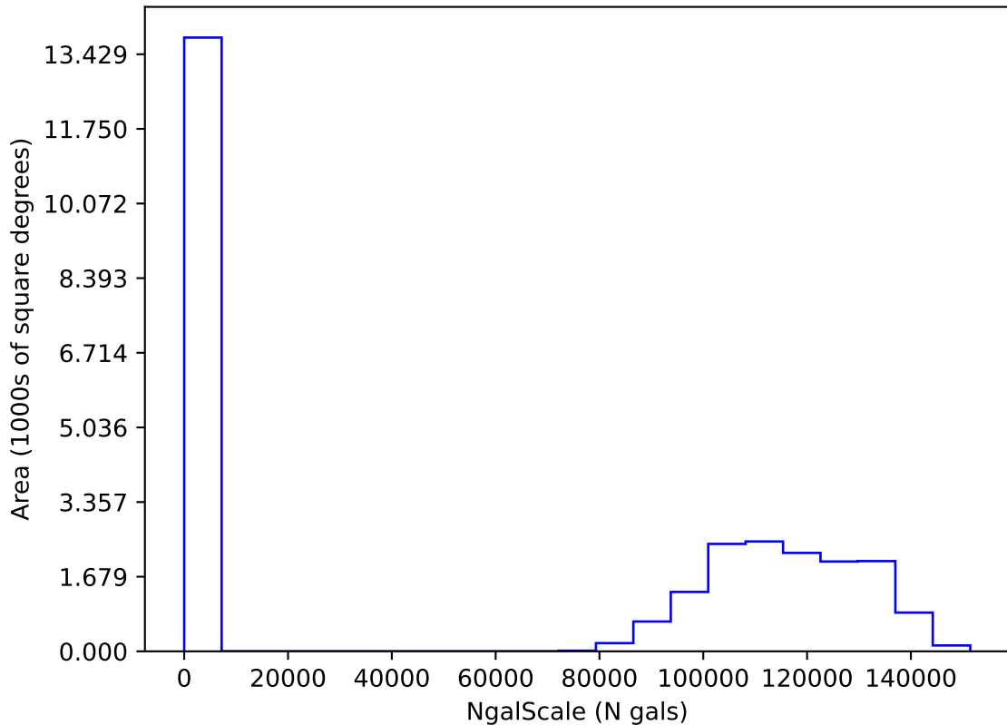
baseline_v3.2_10yrs i: NgalScale
