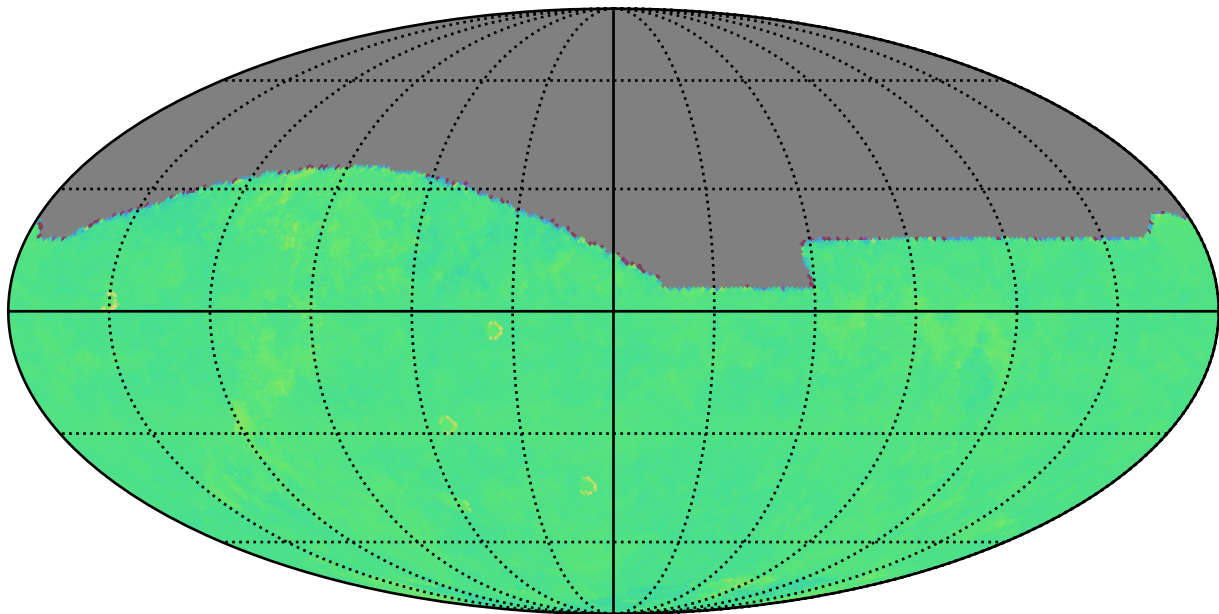
baseline_v3.2_10yrs z: Kuiper rotTelPos
