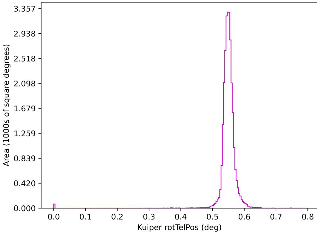
baseline_v3.2_10yrs z: Kuiper rotTelPos
