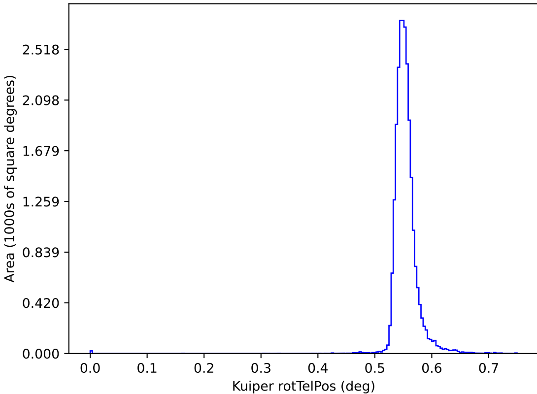
baseline_v3.2_10yrs y: Kuiper rotTelPos
