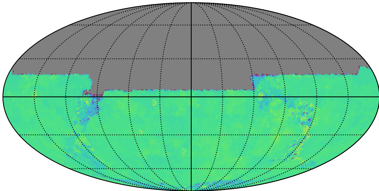
baseline_v3.2_10yrs u: Kuiper rotTelPos
