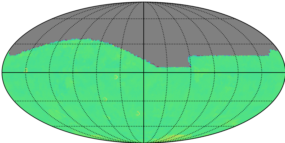
baseline_v3.2_10yrs r: Kuiper rotTelPos
