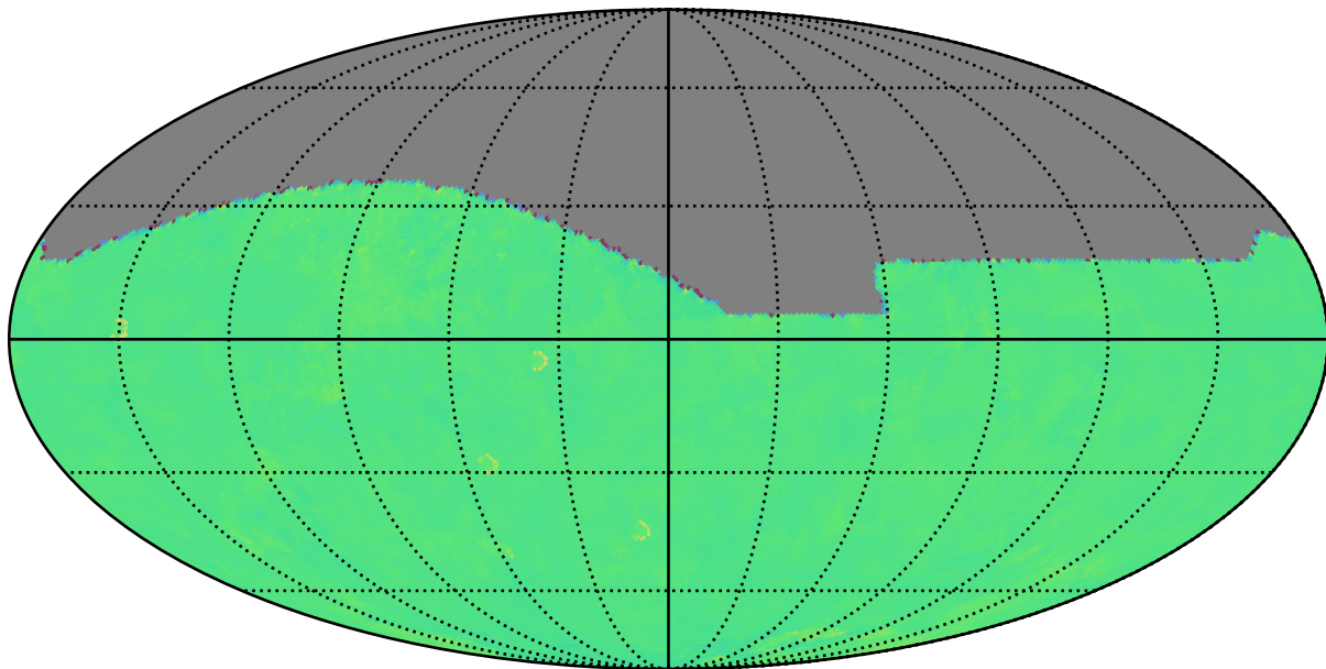
baseline_v3.2_10yrs i: Kuiper rotTelPos
