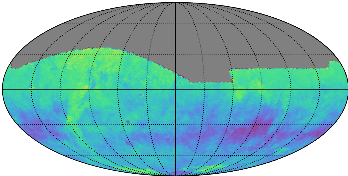
baseline_v3.2_10yrs z: Kuiper rotSkyPos
