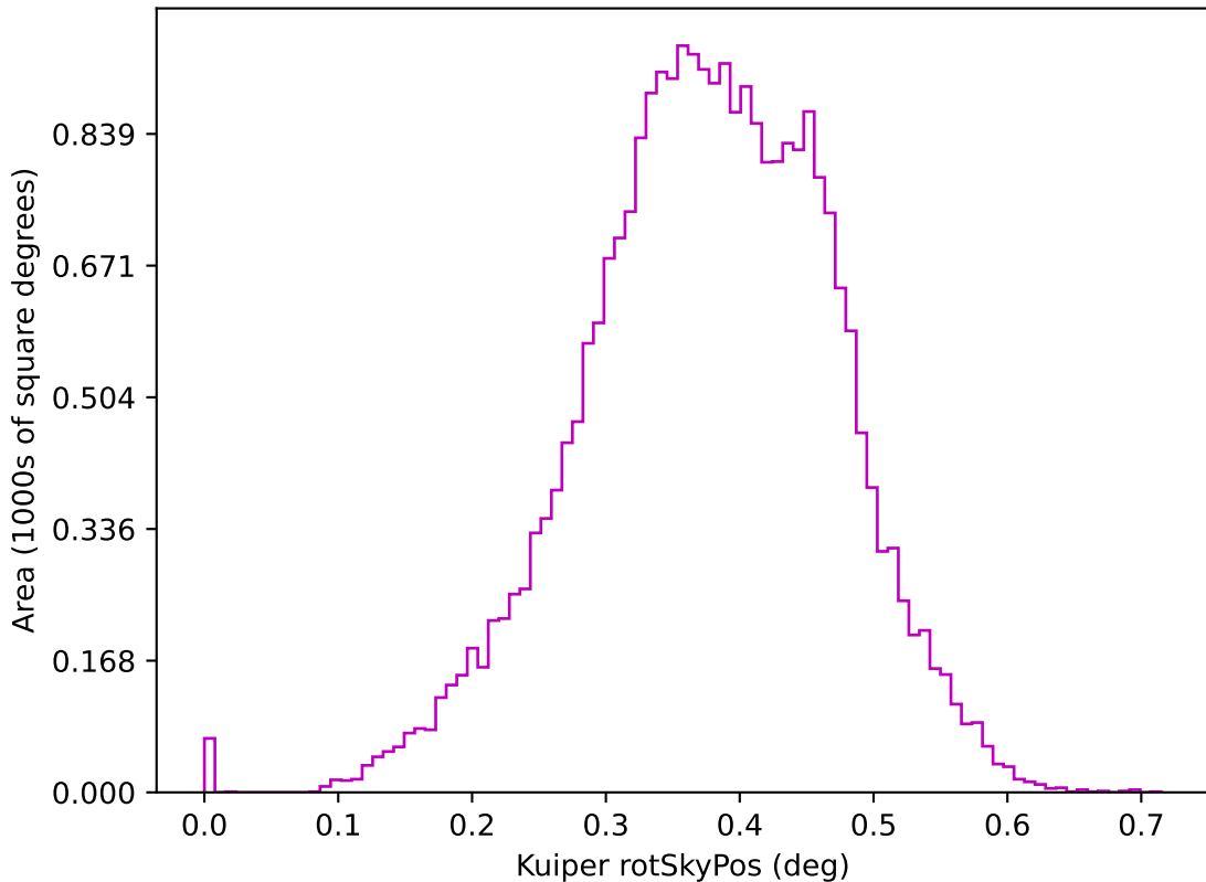
baseline_v3.2_10yrs z: Kuiper rotSkyPos
