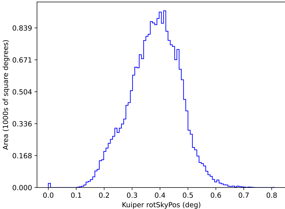
baseline_v3.2_10yrs y: Kuiper rotSkyPos
