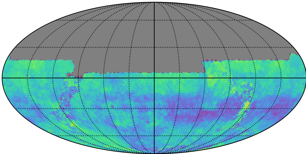
baseline_v3.2_10yrs u: Kuiper rotSkyPos
