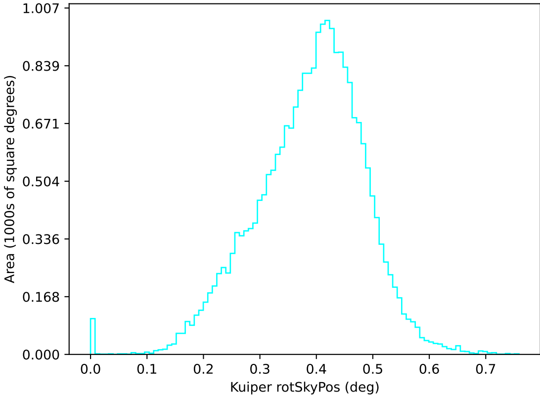
baseline_v3.2_10yrs u: Kuiper rotSkyPos
