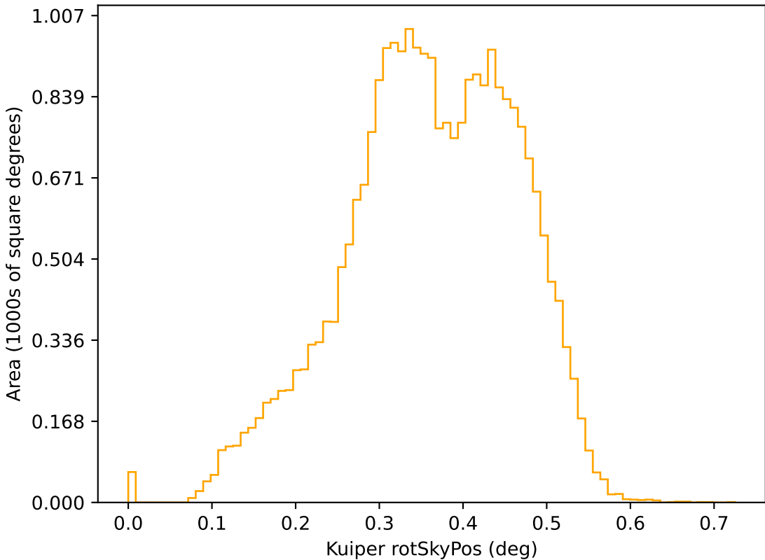
baseline_v3.2_10yrs r: Kuiper rotSkyPos
