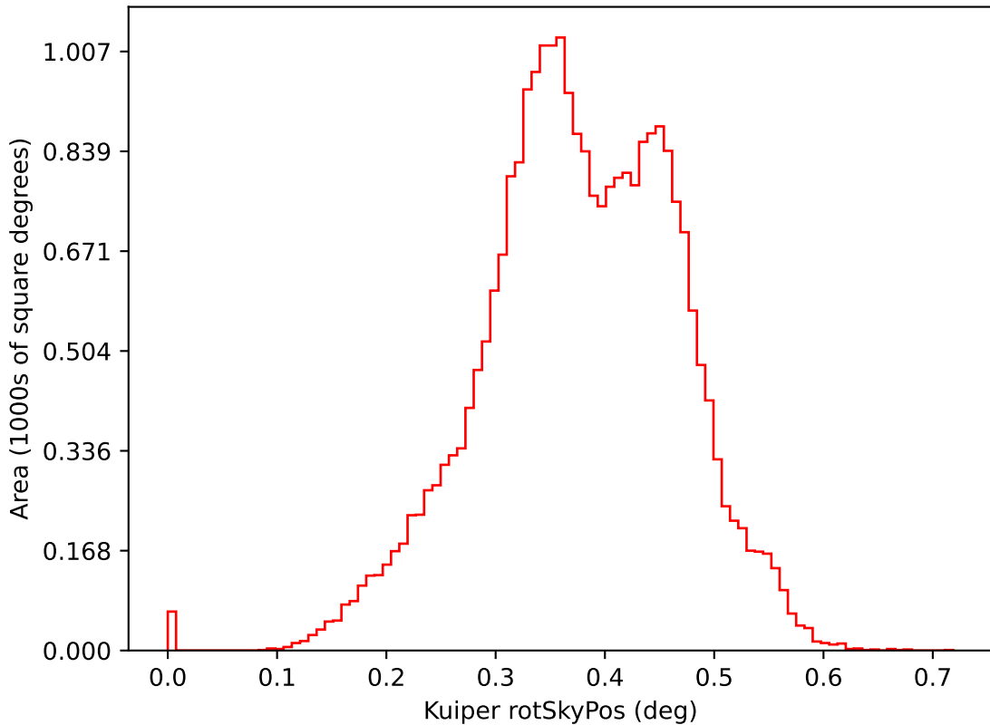
baseline_v3.2_10yrs i: Kuiper rotSkyPos
