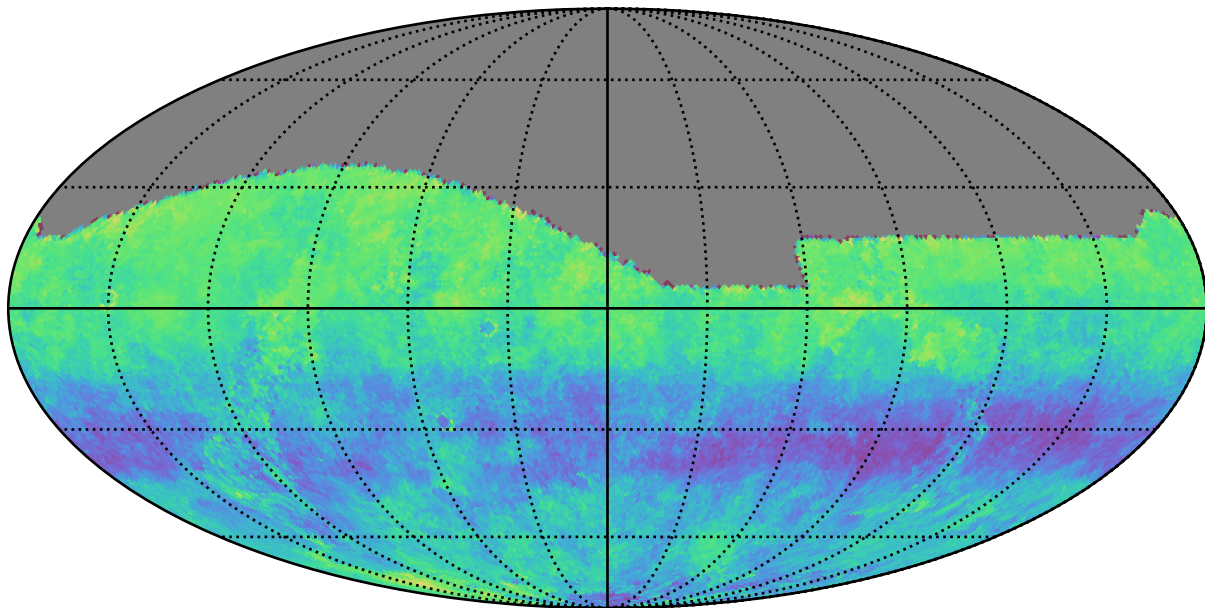
baseline_v3.2_10yrs g: Kuiper rotSkyPos
