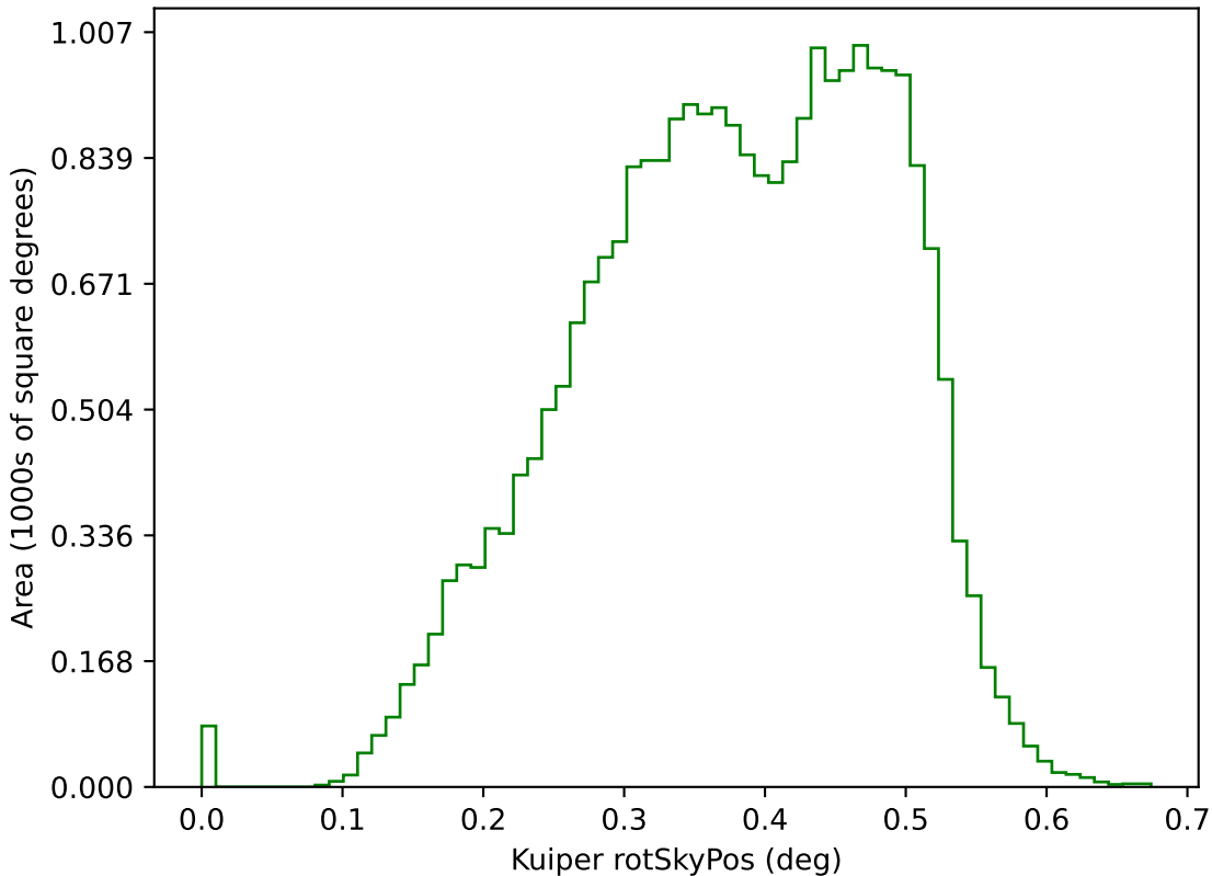
baseline_v3.2_10yrs g: Kuiper rotSkyPos
