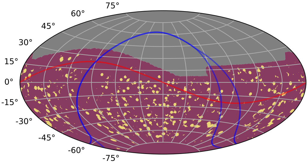
baseline_v3.2_10yrs all models: KNePopMetric_all_multi_detect
